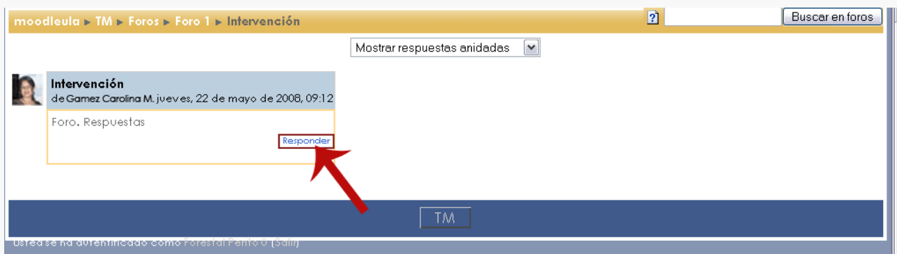
Imagen 3
