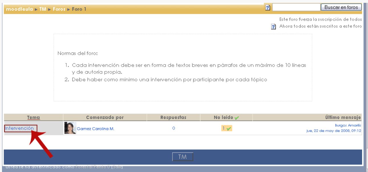
Imagen 2
